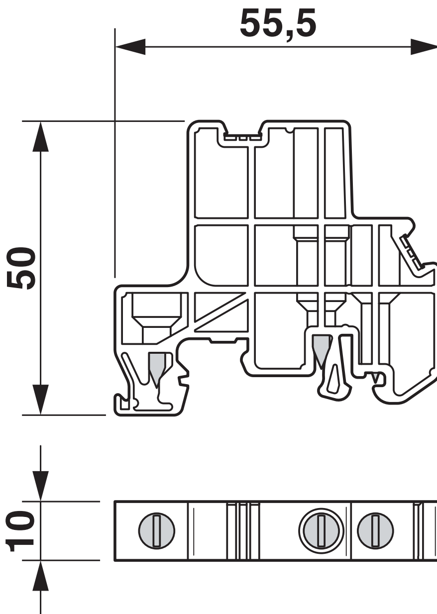
Rysunek wymiarowy
