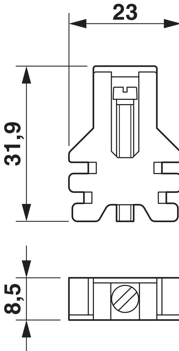
Rysunek wymiarowy
