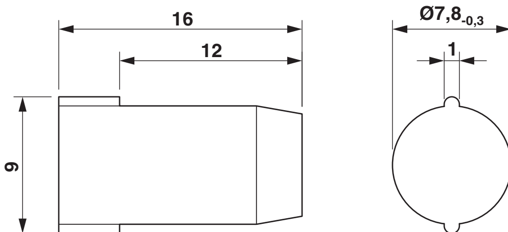
Rysunek wymiarowy
