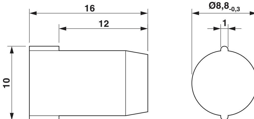
Rysunek wymiarowy
