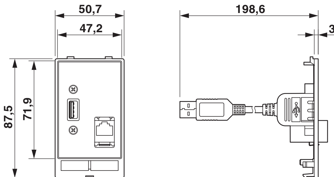
Rysunek wymiarowy
