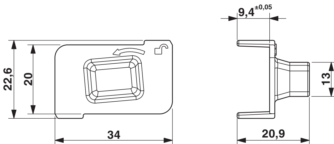
Rysunek wymiarowy
