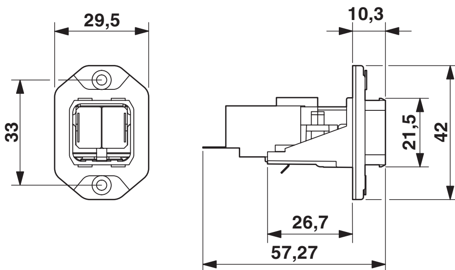
Rysunek wymiarowy
