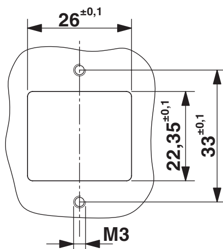
Rysunek wymiarowy
