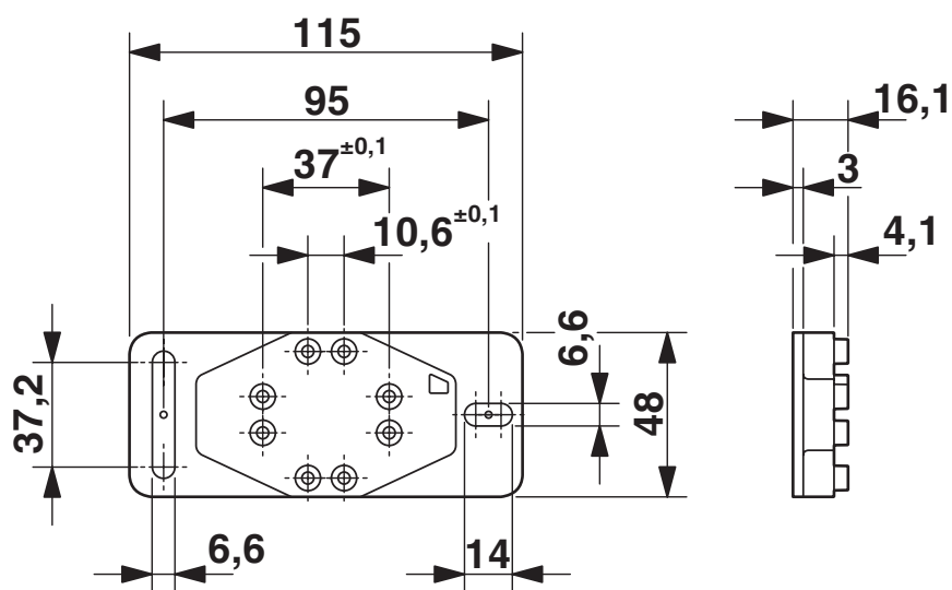
Rysunek wymiarowy
