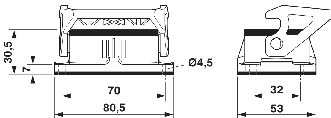
Rysunek wymiarowy
