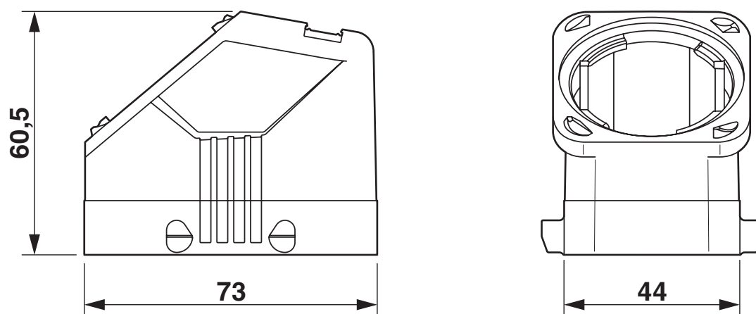
Rysunek wymiarowy
