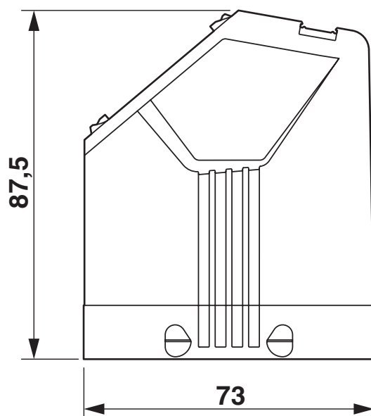
Rysunek wymiarowy
