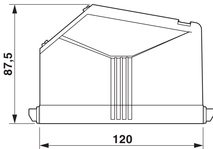
Rysunek wymiarowy
