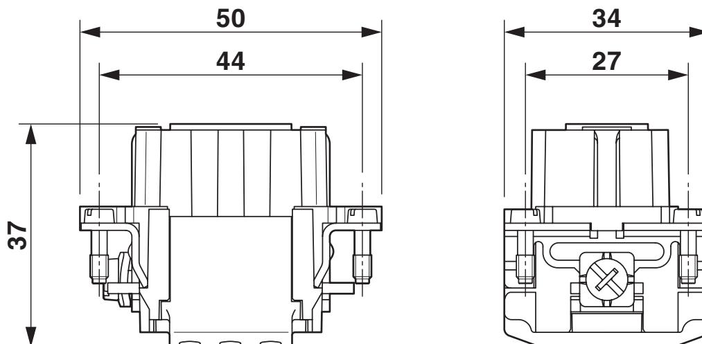
Rysunek wymiarowy
