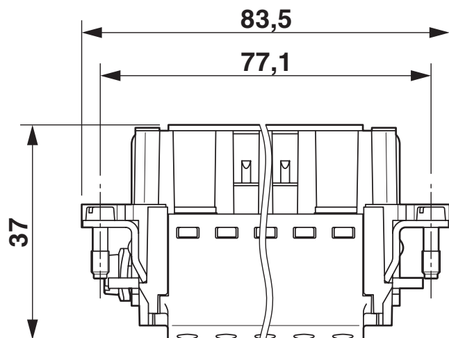
Rysunek wymiarowy
