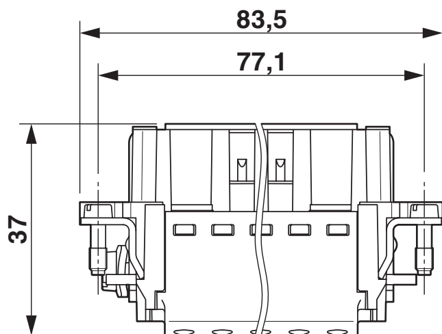
Rysunek wymiarowy
