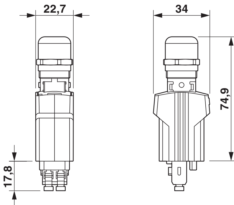
Rysunek wymiarowy
