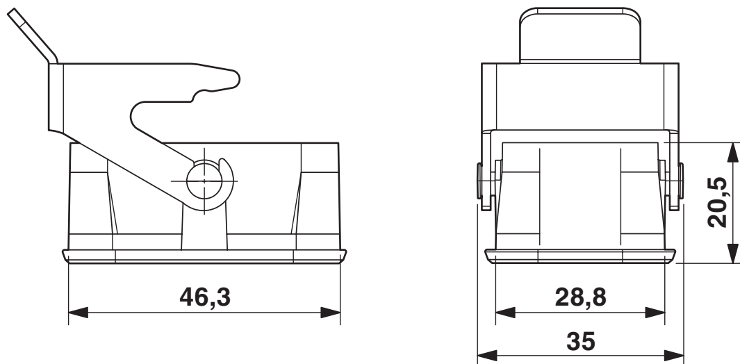
Rysunek wymiarowy
