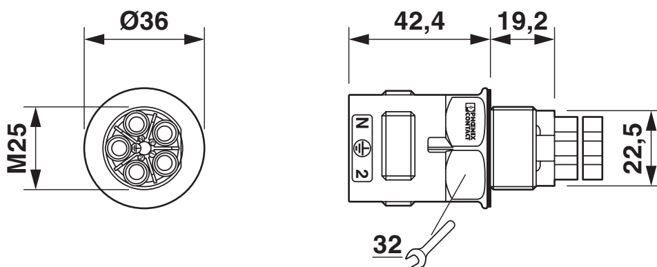
Rysunek wymiarowy QPD W 4PE6,0 M25
