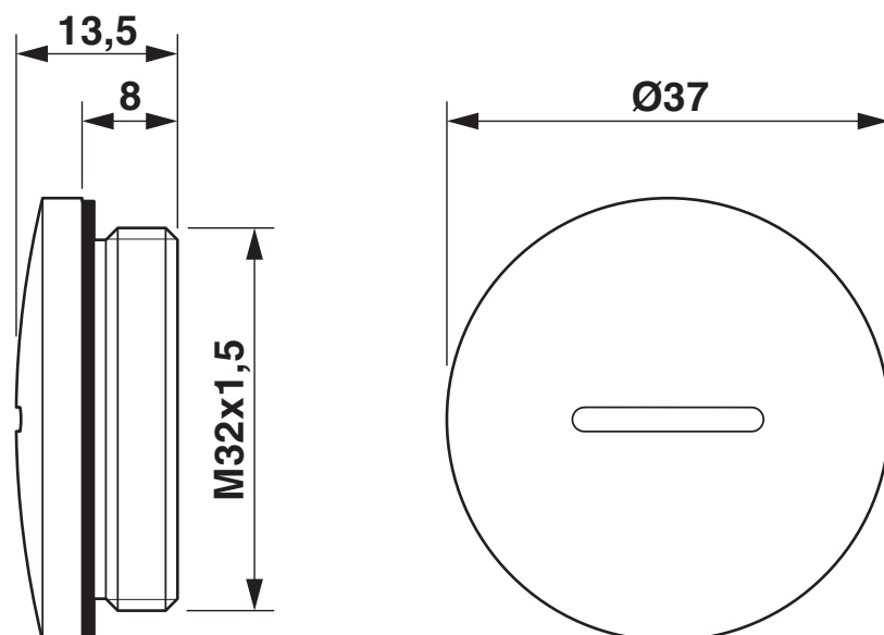
Rysunek wymiarowy
