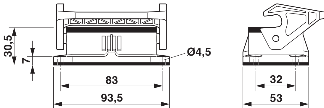
Rysunek wymiarowy
