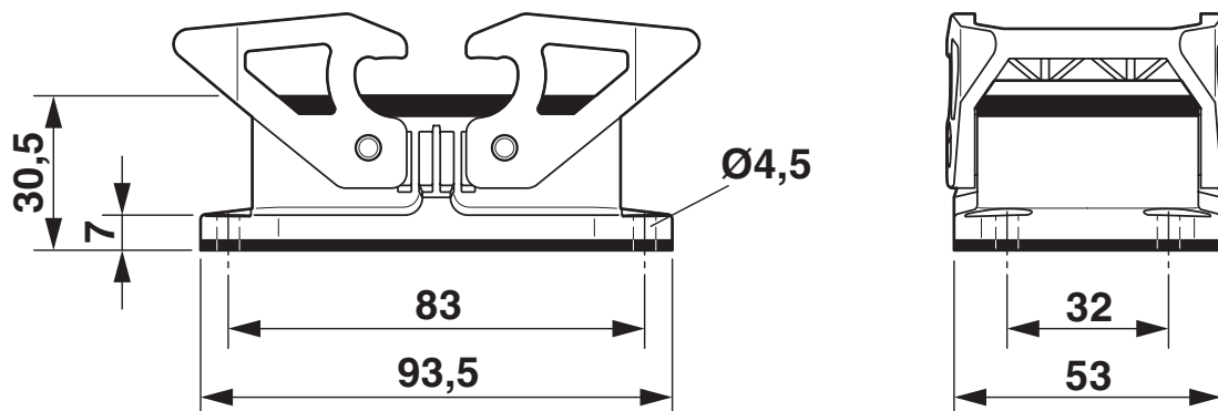
Rysunek wymiarowy
