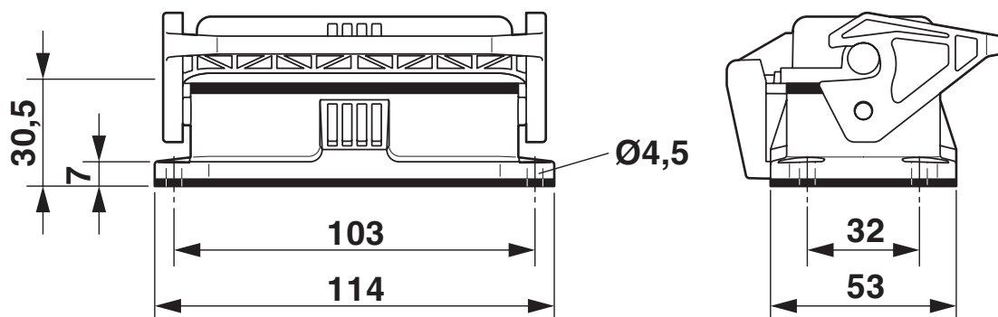
Rysunek wymiarowy
