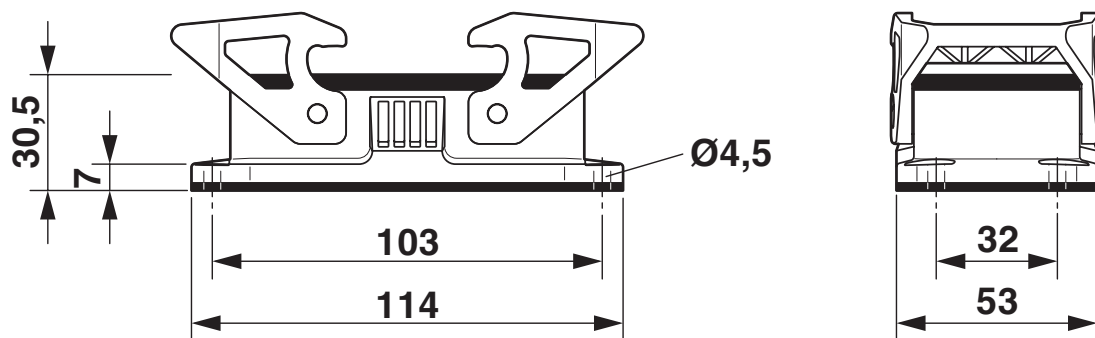
Rysunek wymiarowy
