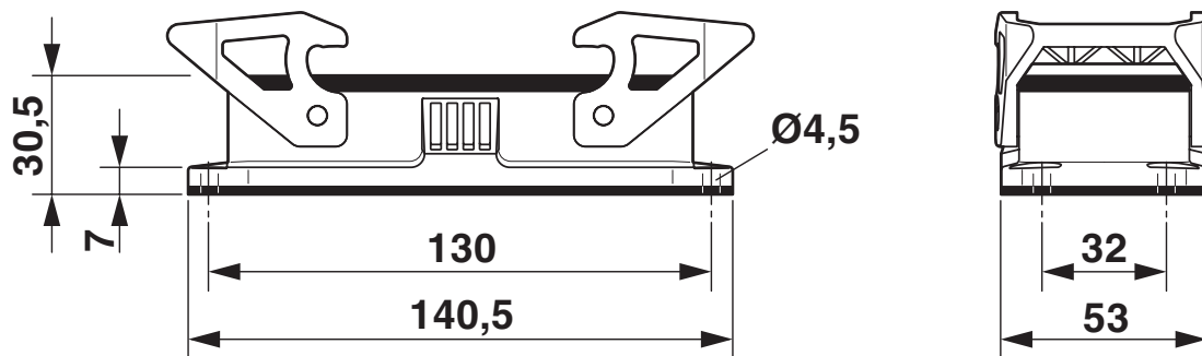
Rysunek wymiarowy
