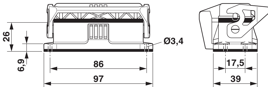
Rysunek wymiarowy
