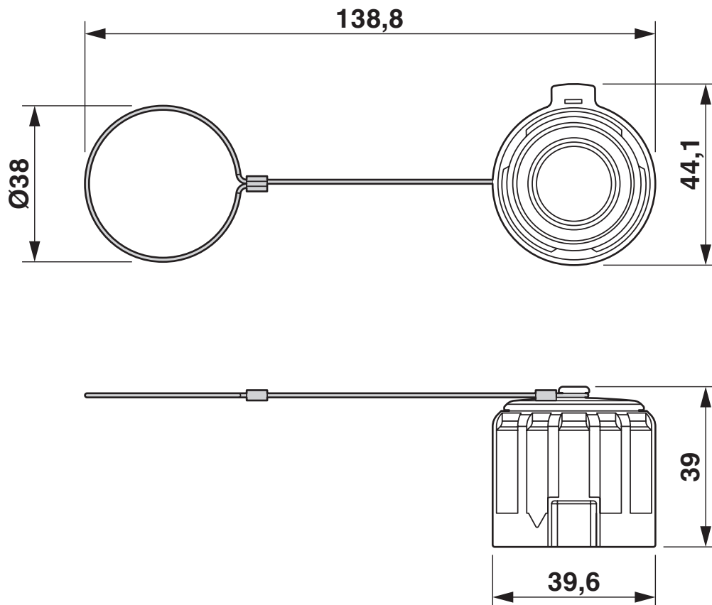
Rysunek wymiarowy
