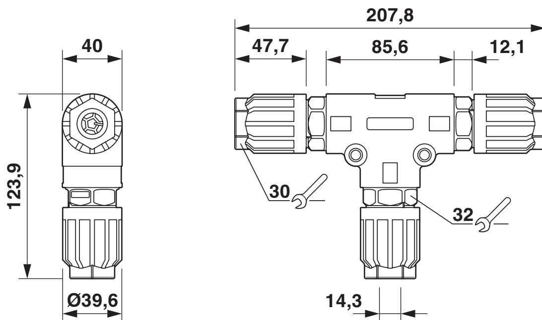
Rysunek wymiarowy
