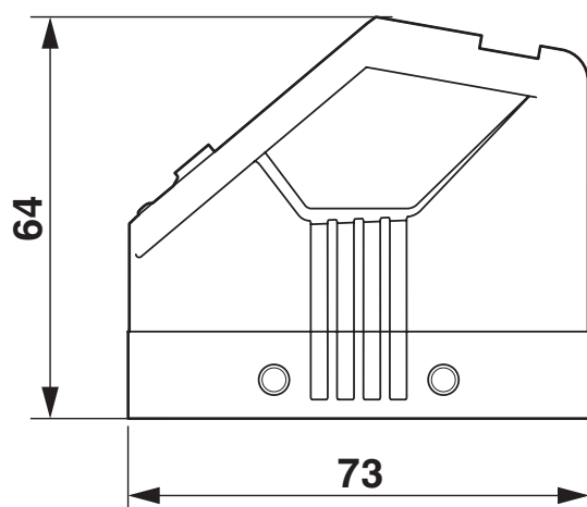
Rysunek wymiarowy
