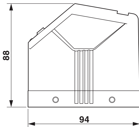
Rysunek wymiarowy
