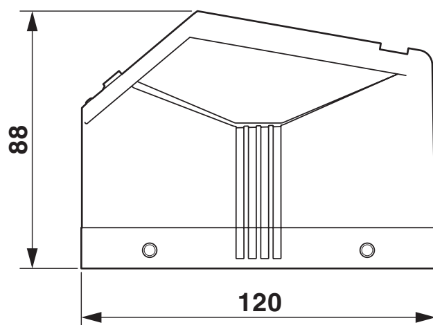
Rysunek wymiarowy
