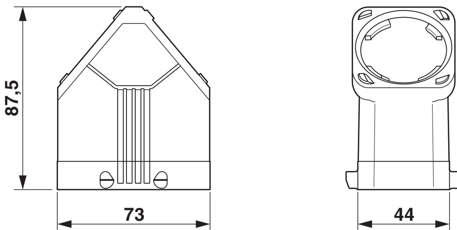
Rysunek wymiarowy
