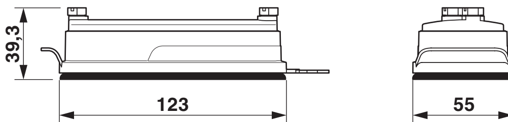
Rysunek wymiarowy
