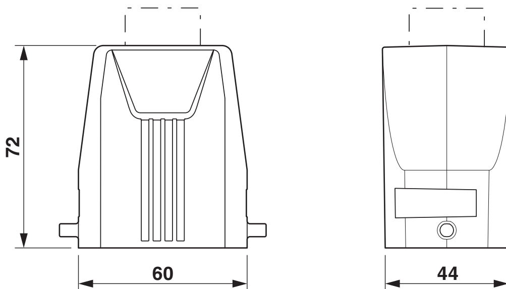
Rysunek wymiarowy
