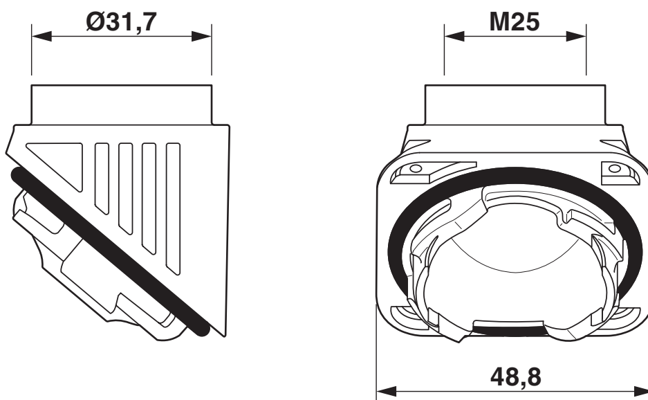
Rysunek wymiarowy
