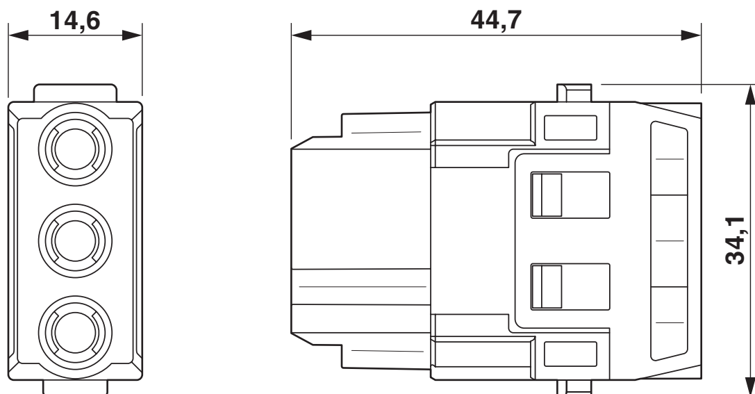
Rysunek wymiarowy
