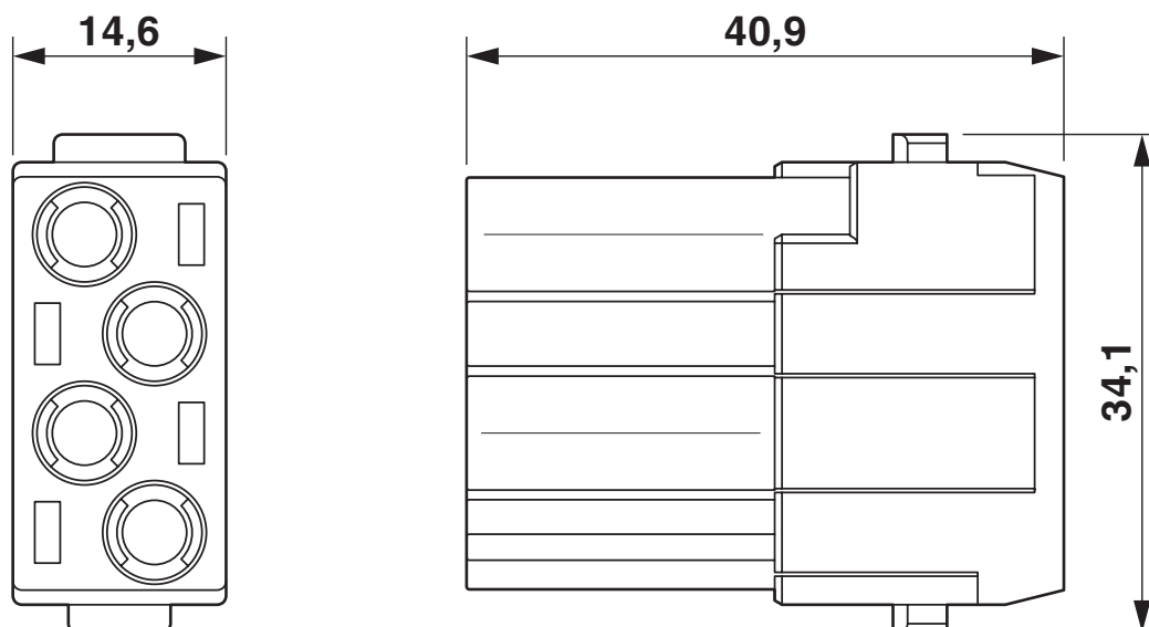
Rysunek wymiarowy
