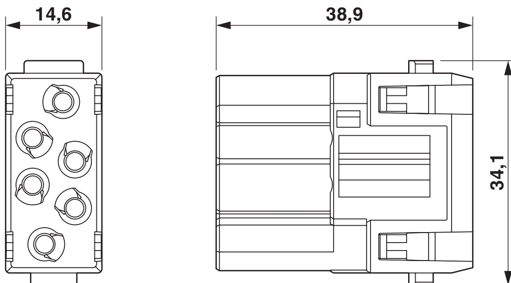
Rysunek wymiarowy
