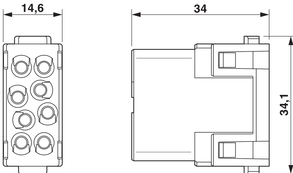
Rysunek wymiarowy
