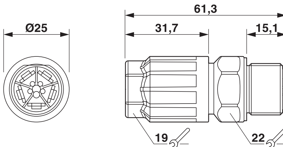
Rysunek wymiarowy
