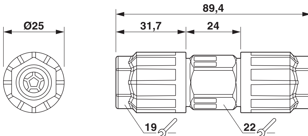
Rysunek wymiarowy
