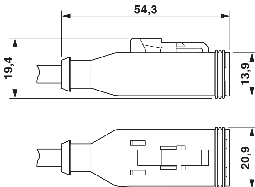
Rysunek wymiarowy
