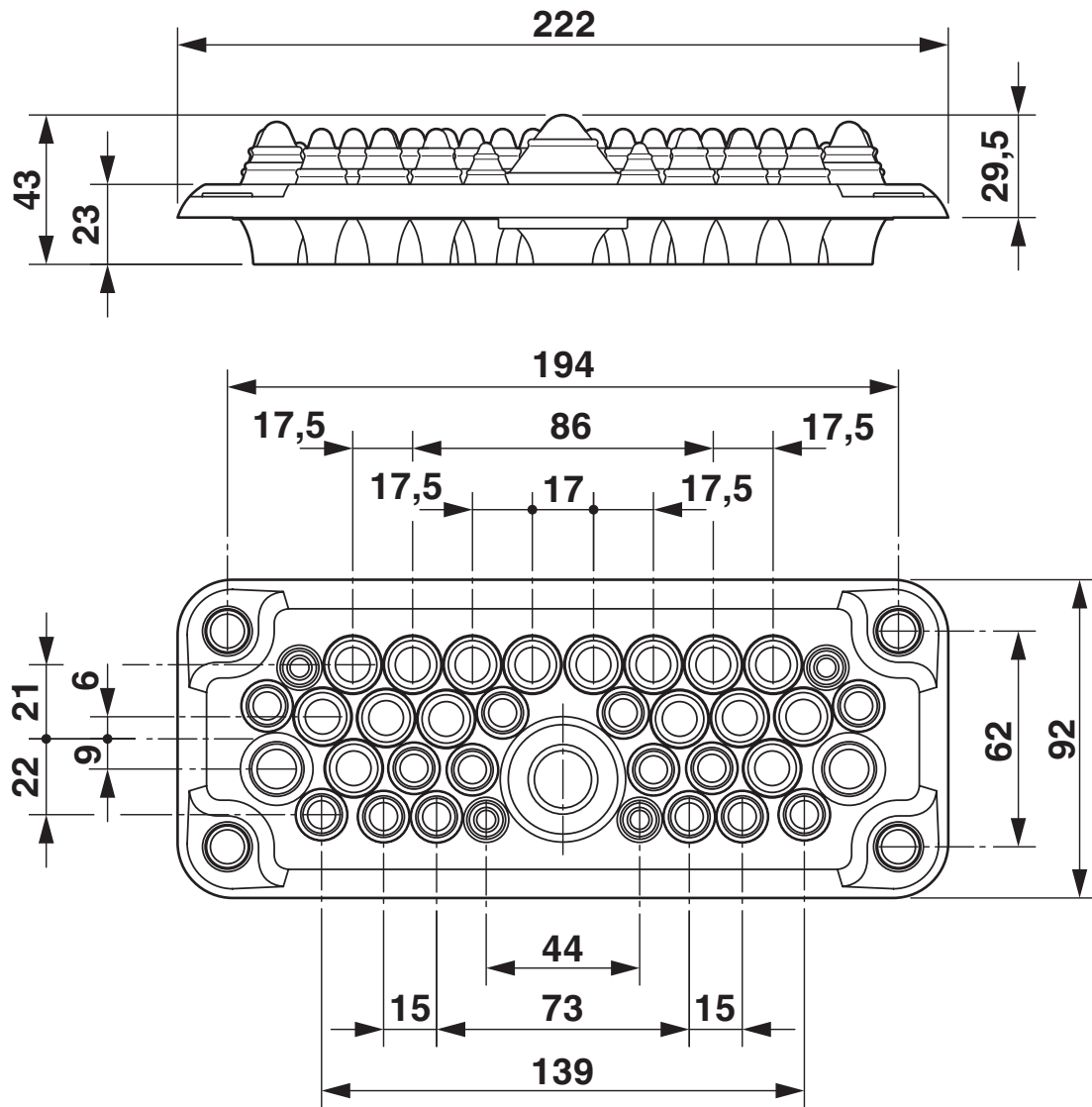
Rysunek wymiarowy
