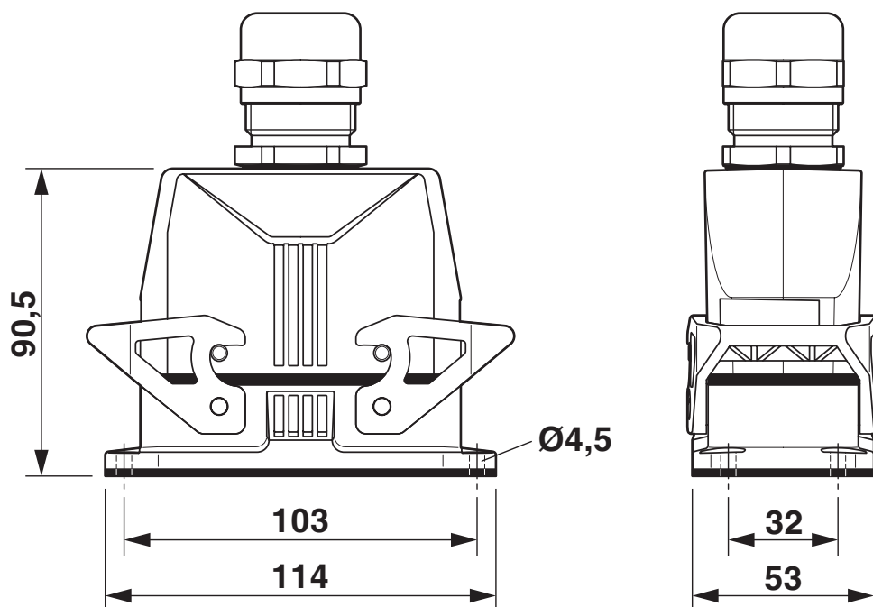
Rysunek wymiarowy
