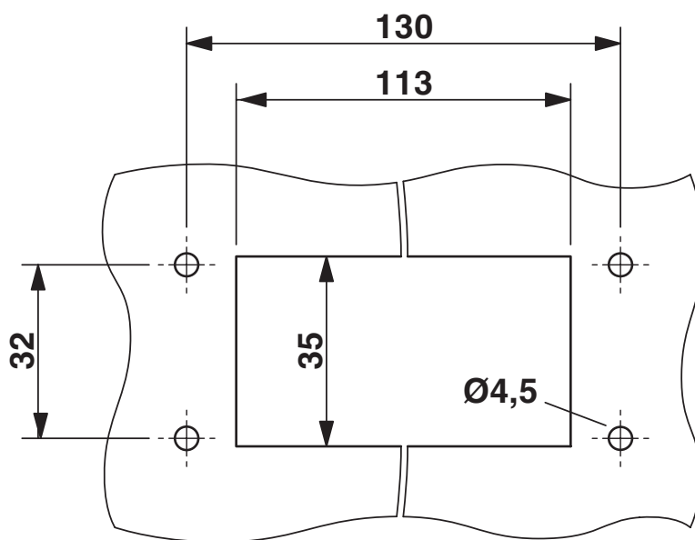
Rysunek wymiarowy
