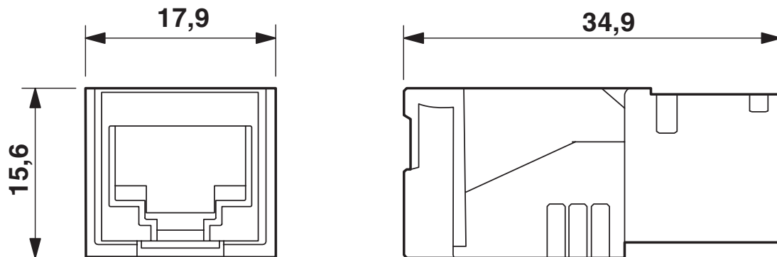
Wkładka żeńska RJ45
