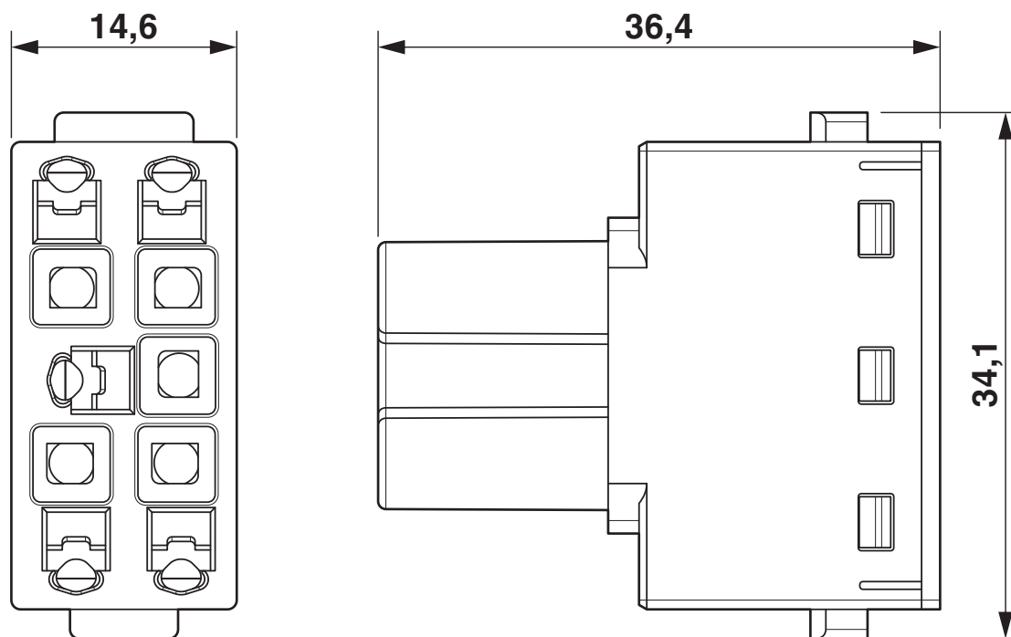
Rysunek wymiarowy
