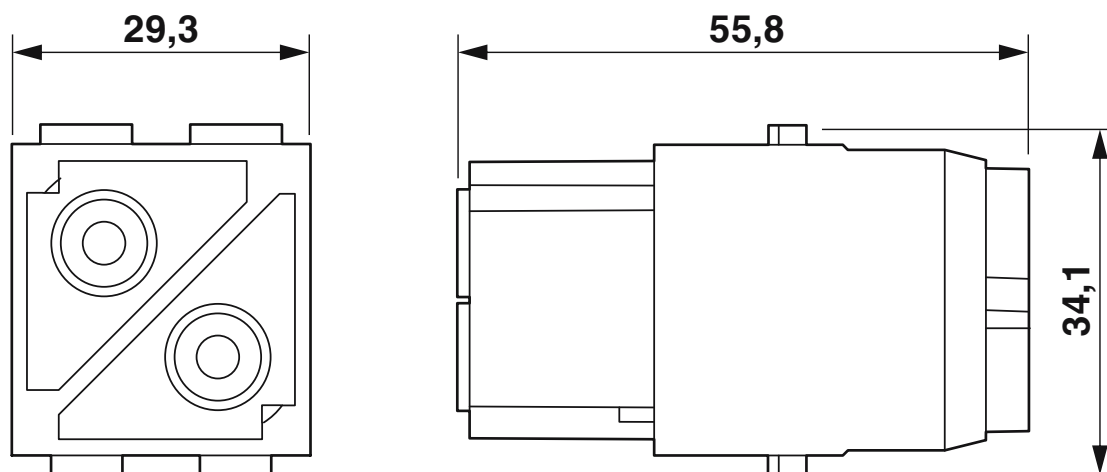
Moduł wtyków żeńskich
