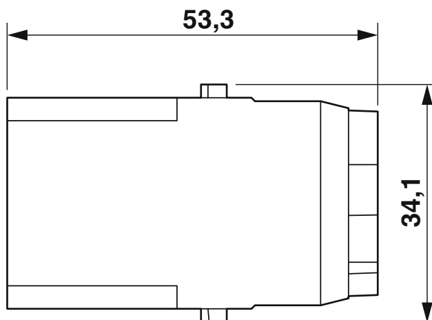
Rysunek wymiarowy
