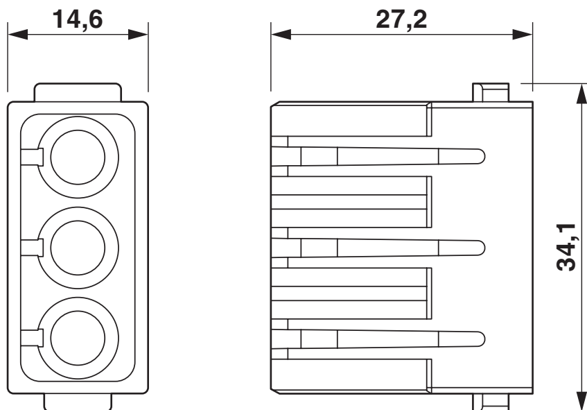
Rysunek wymiarowy
