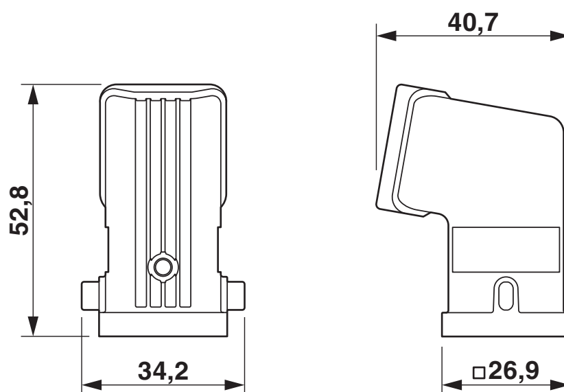
Rysunek wymiarowy
